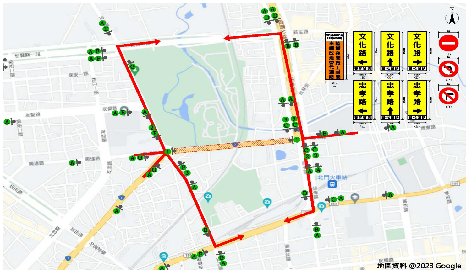
博愛陸橋限高架施工設施佈設及替代道路規劃示意圖
